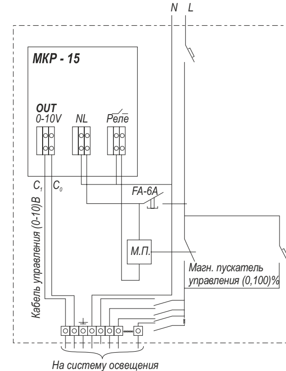
Схема подключения АСУ-ОП “Ника”
